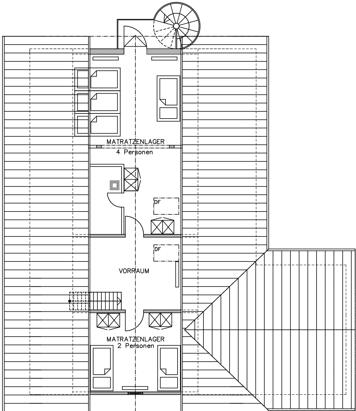
DACHGESCHOSS – SCHWARZSCHNIEDERHOF
